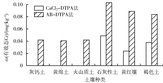
图 3 AB-DTPA 法和 \text{CaCl}_2 - \text{DTPA} 法提取土壤中有有效态 Cr 的比较
